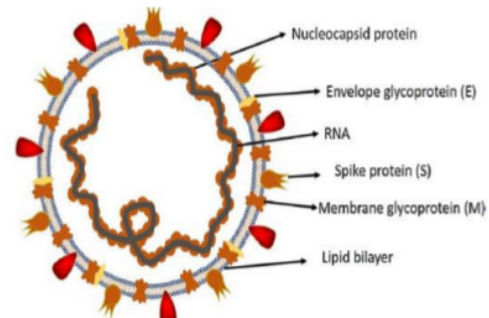
Gambar 1. Struktur coronavirus (14).
