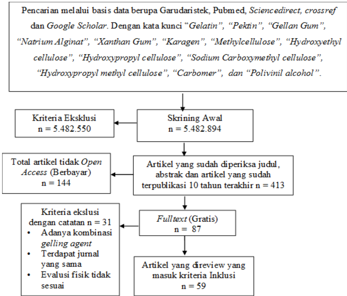
Gambar 1. Diagram alir penyusunan literatur
