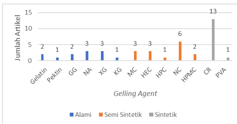
Gambar 2. Jumlah Artikel Gelling Agent Jenis Polimer ( n = 41 )
